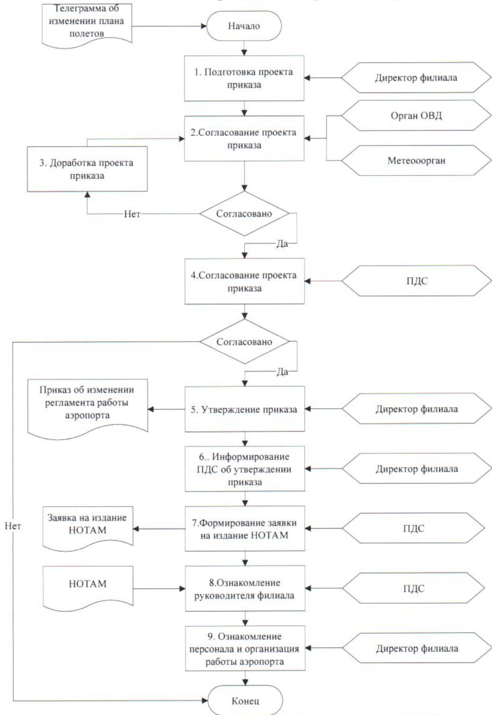
Схема изменения регламента работы аэропорта
